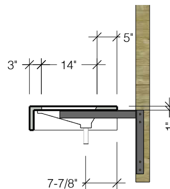
Coupe A-A
